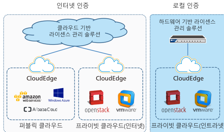
그림 1. Hillstone LMS 솔루션
